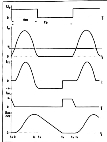
2. ábra, A kvázirezonáns konverter jellemző jelalakjai
