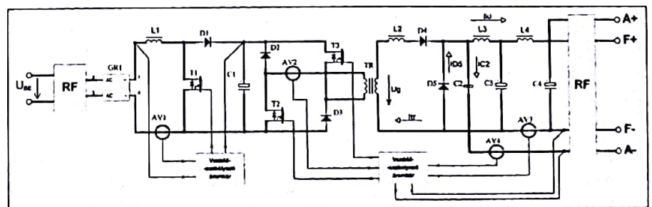
1. ábra. A HPQ 230/48-7,5 típusú akkumulátortöltő elvi felépítése
